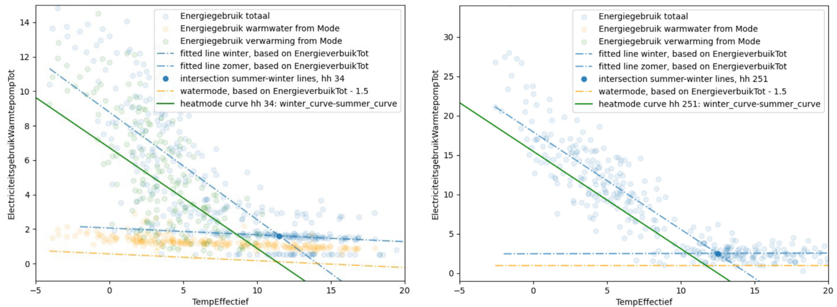
Figuur 6: twee grafieken die de weergevoeligheid van twee woningen schetst
