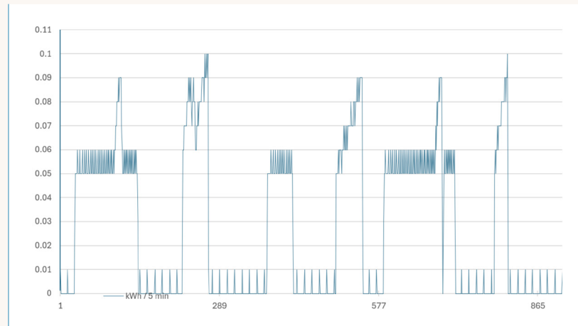
Figuur 7: verbruikspatroon van een warmtepomp gedurende drie dagen (tijdsresolutie 5 minuten)
