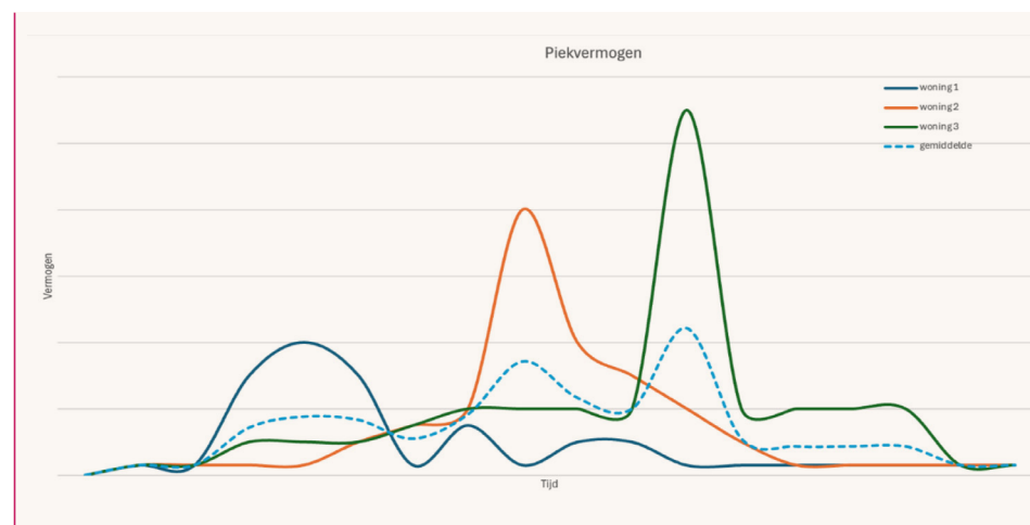
Figuur 1: Relatie tussen de gevraagde vermogens van individuele woningen (dichte lijnen) en het gelijktijdige gevraagde vermogen van de drie woningen gemiddeld (stippellijn).
