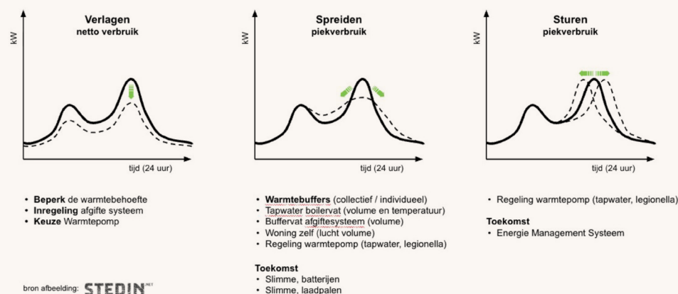
Figuur 3: drie mogelijke routes om netbelasting te verlagen (bron: Stedin)
