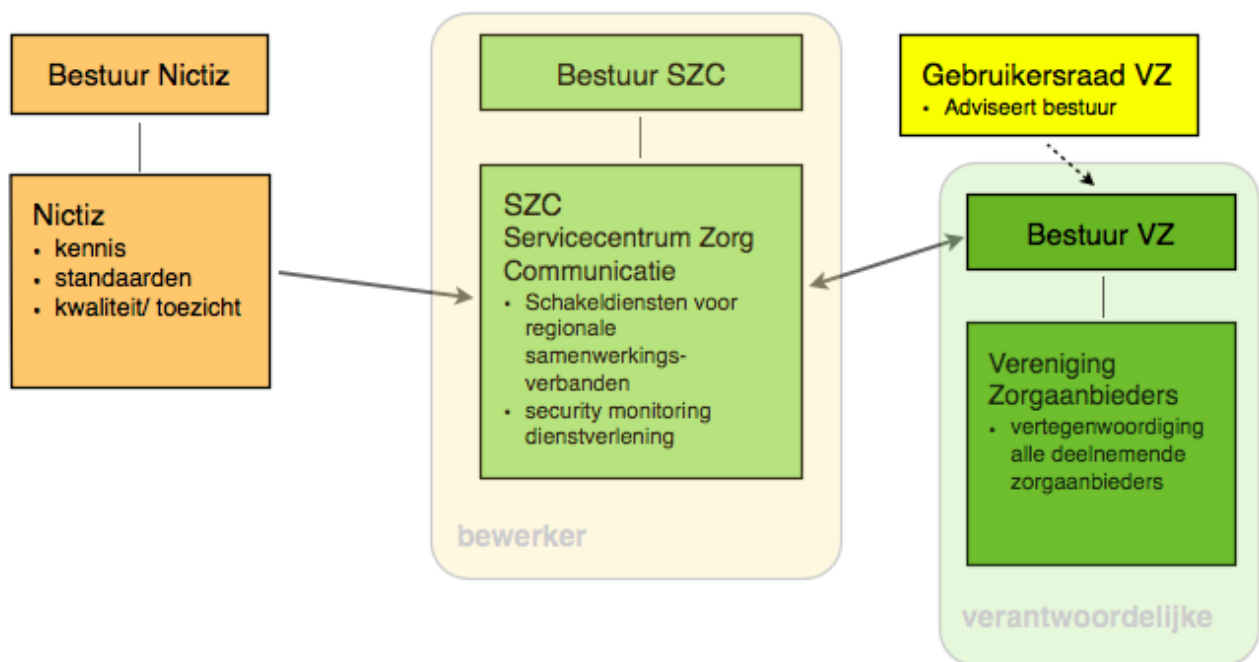
Figuur 1. Doorstartmodel
